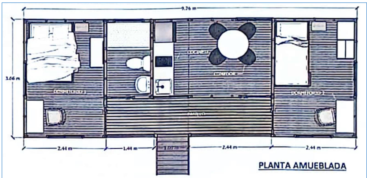
Diagrama 1: Propuesta arquitectónica módulo de cuarto a construir – Estación Biológica Hector Centeno
